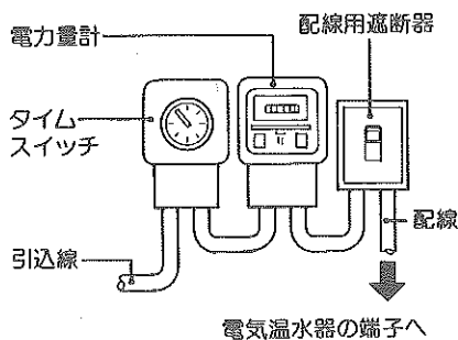
電源ボックスカバーの内部
