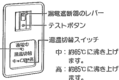
電源ボックスカバーの内部
